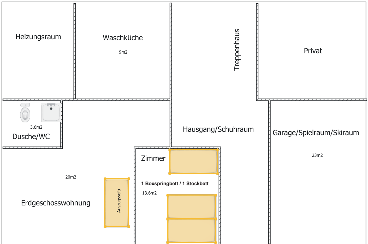
Chalet Viola, Grundrissplan Wohnung Erdgeschoss
